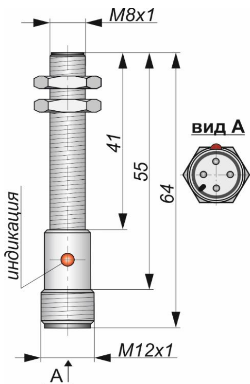
Габаритный чертеж
