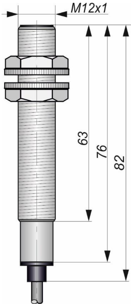
Габаритный чертеж
