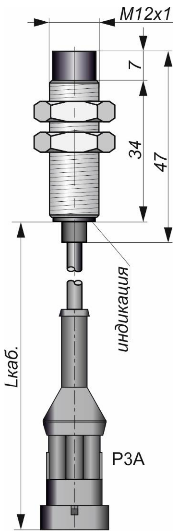
Габаритный чертеж
