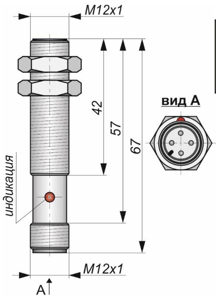
Габаритный чертеж
