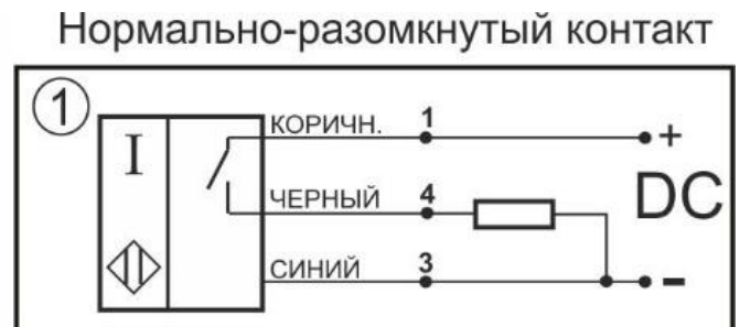
Схема соединения
