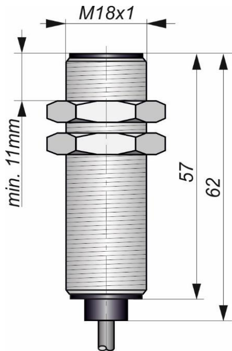
Габаритный чертеж
