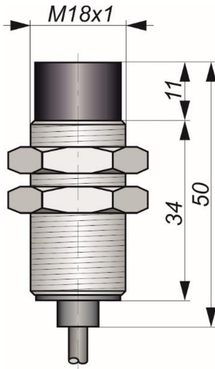
Габаритный чертеж
