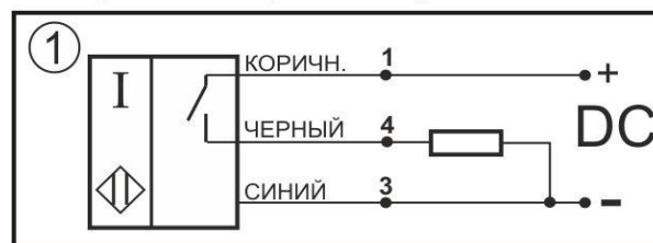
Схема подключения Нормально-разомкнутый контакт
