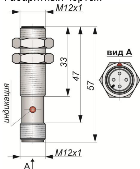
Габаритный чертеж
