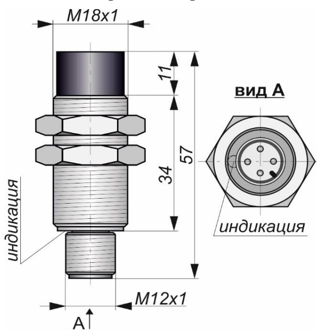
Габаритный чертеж
