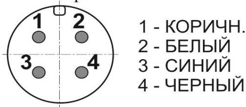
Цоколевка разъема
