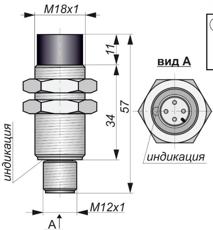
Габаритный чертеж
