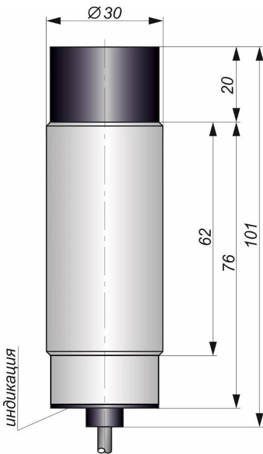
Габаритный чертеж
