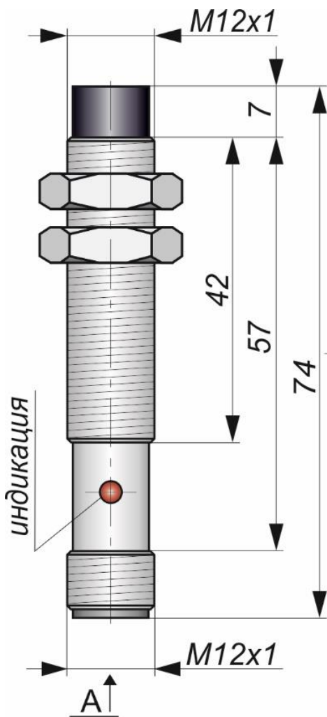
Габаритный чертеж
