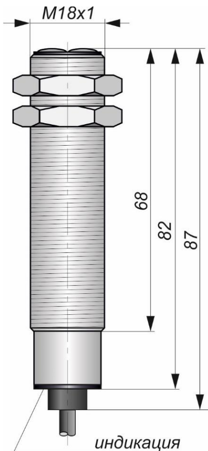
Габаритный чертеж
