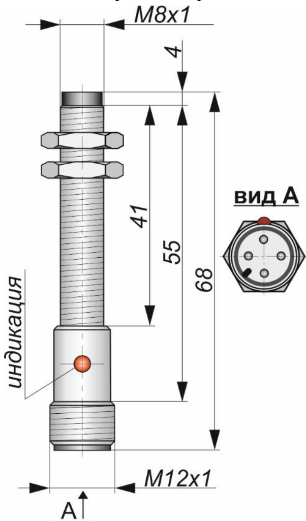
Габаритный чертеж
